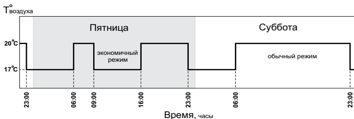
Рис.7 График температуры воздуха в помещении для Режима 3.
